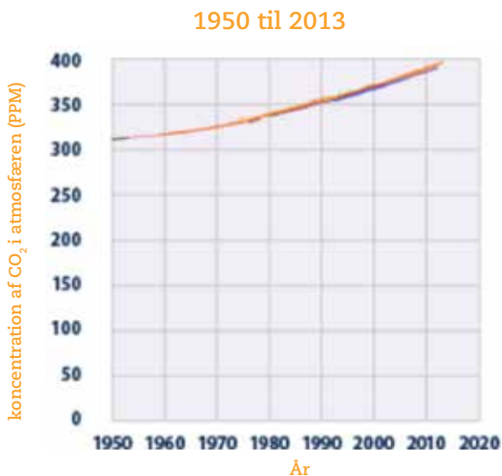
Fig. 2. Koncentration af CO 2 i atmosfæren 1950-2013. Kilde: EPA
